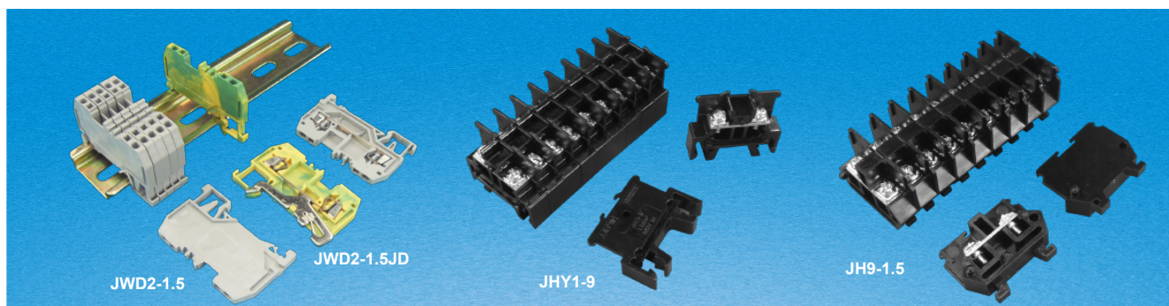
弹片固定结构 Shrapnel fixed construction
